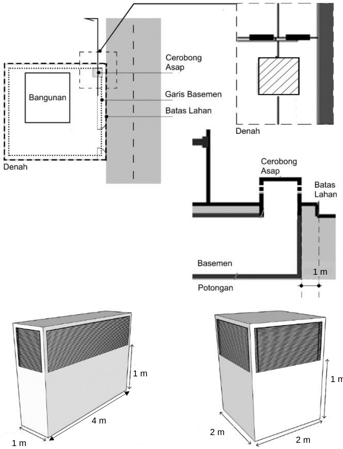
Contoh: beberapa konfigurasi luas cerobong asap sebesar 4 m 2
